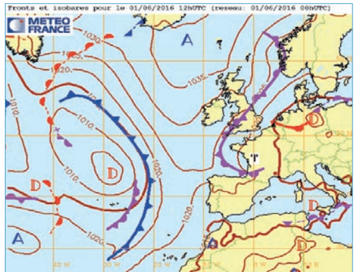
Cette carte présente la frontologie et la pression au niveau de la mer à grande échelle (proche-atlantique) à 12 h ou 24 h d'échéance, et ne peut pas se superposer sur un TEMSI.
